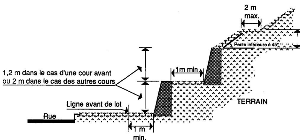
Croquis 9.1 Hauteur d'un mur de soutènement
