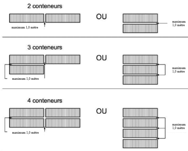
Croquis 7.1 Implantation de plusieurs conteneurs
