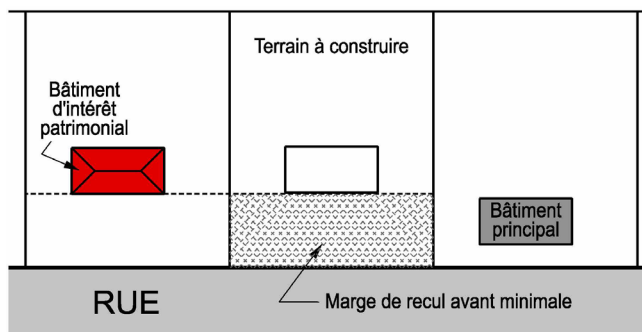
Croquis 6.3 Implantation d'un bâtiment principal adjacent à un bâtiment d'intérêt patrimonial
